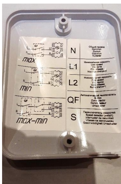
Bekötési rajz
